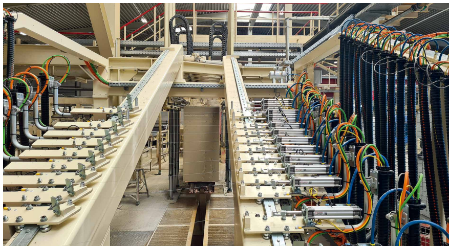
现代化升级之前（左侧）与之后（右侧）。从精准提升到臻精准和灵活：带有自动布线调整的新型厚度切割机
