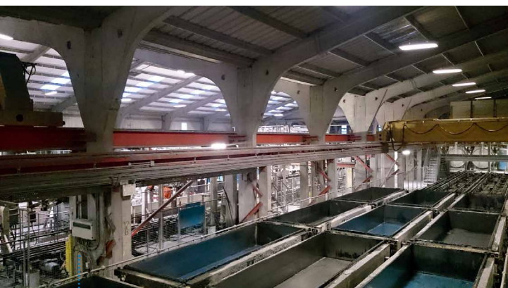
2018年之前的H+H Celcon公司：由Wehrhahn公司建造的旧厂仍在生产优质的加气混凝土，但设备已不再尖端
